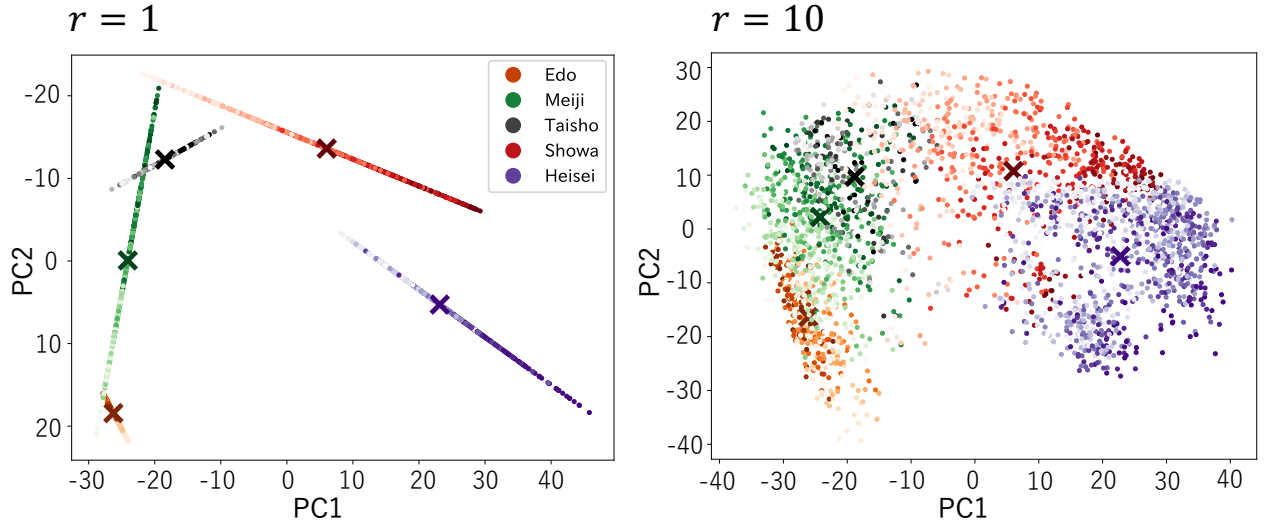
図2 Swallow-13bにおける日本の時系列構造のPCAによる可視化結果. 左は1個の潜在変数 ( r = 1 ) で PLS の逆変換を使った場合の可視化結果であり, 右は10個の潜在変数 ( r = 10 ) で PLS の逆変換を使った場合の可視化結果である.
